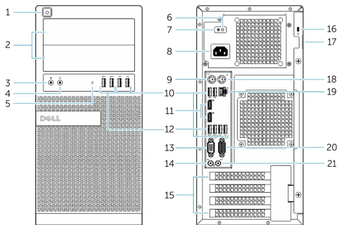
圖 1. 迷你直立型電腦的前視圖與後視圖
